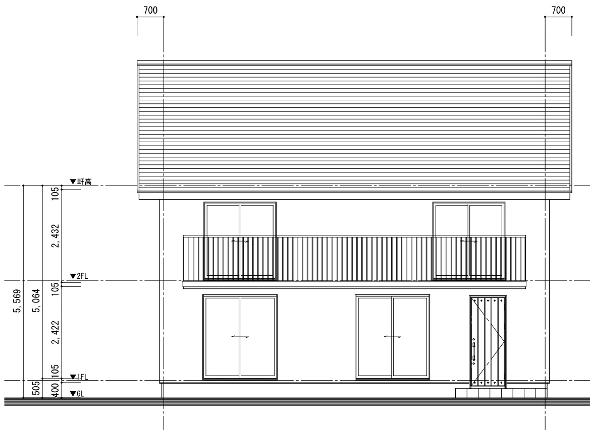
南側立面図
