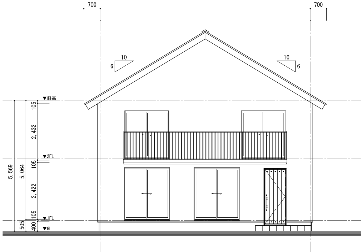
南側立面図
